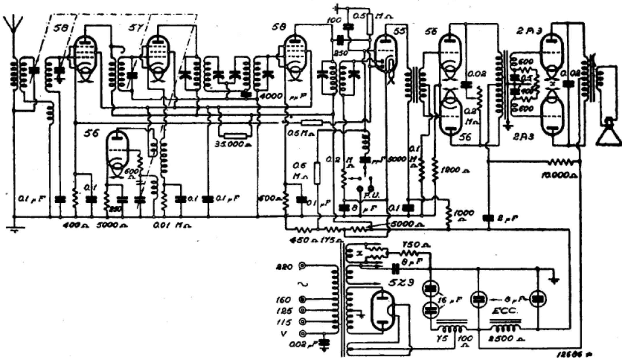
CRESA RADIO . MOD. « SUPERLA JUPITER »
